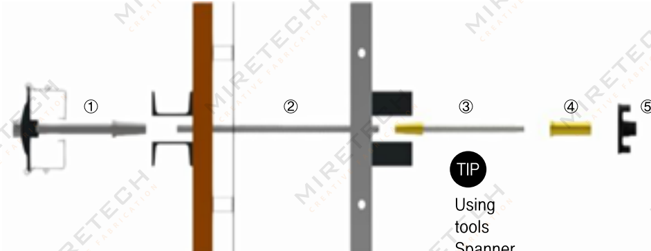
Outer Gang-Form 외부 갱폼
