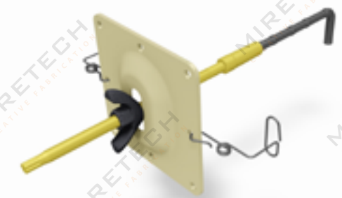
Gang Form Fixing Anchor [Set] [Add] 갱폼 고정용 볼트 [세트] [추가용]
