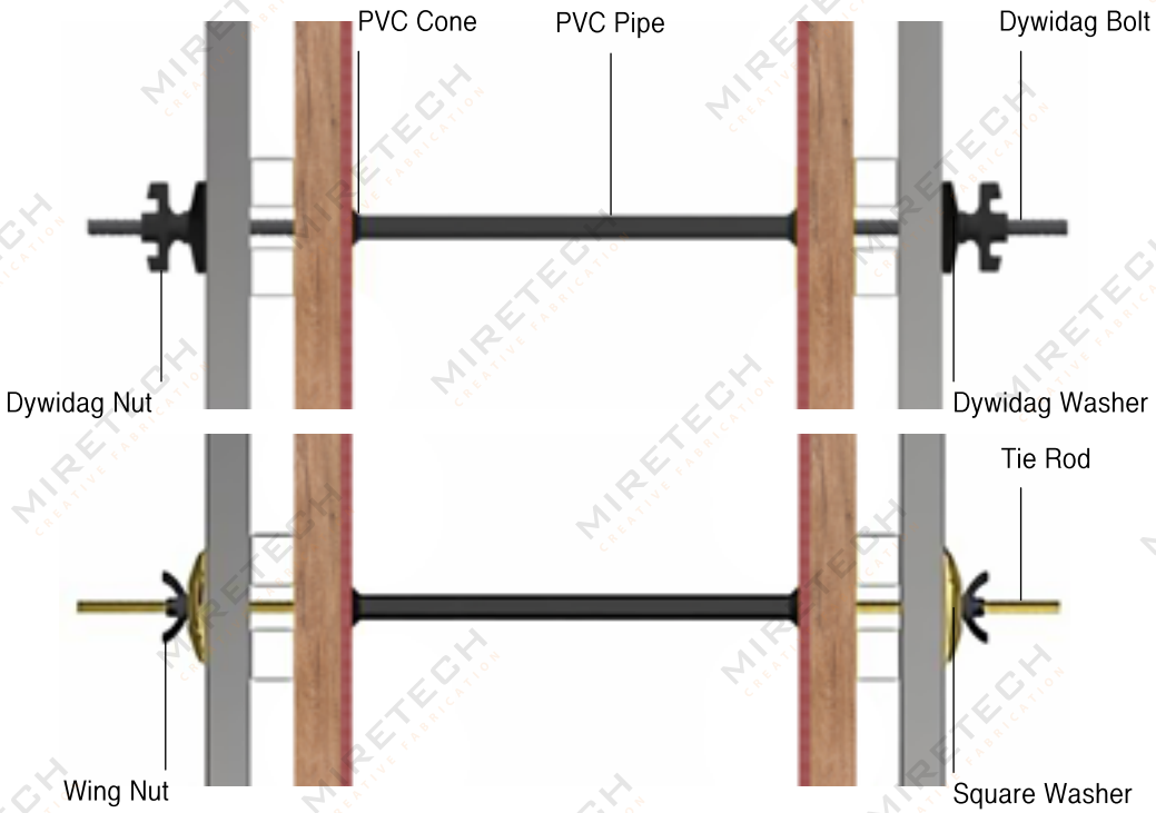
Tie Rod 타이로드 Tensile Load / ½" 4,500kgf, 5/8" 7,000kgf
