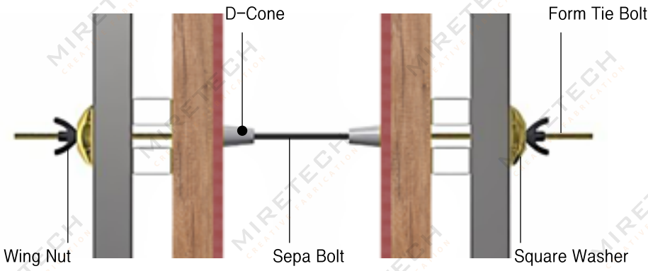
Sepa Bolt 세파 볼트 Tensile Load / ½" 4,500kgf, 5/8" 7,000kgf
